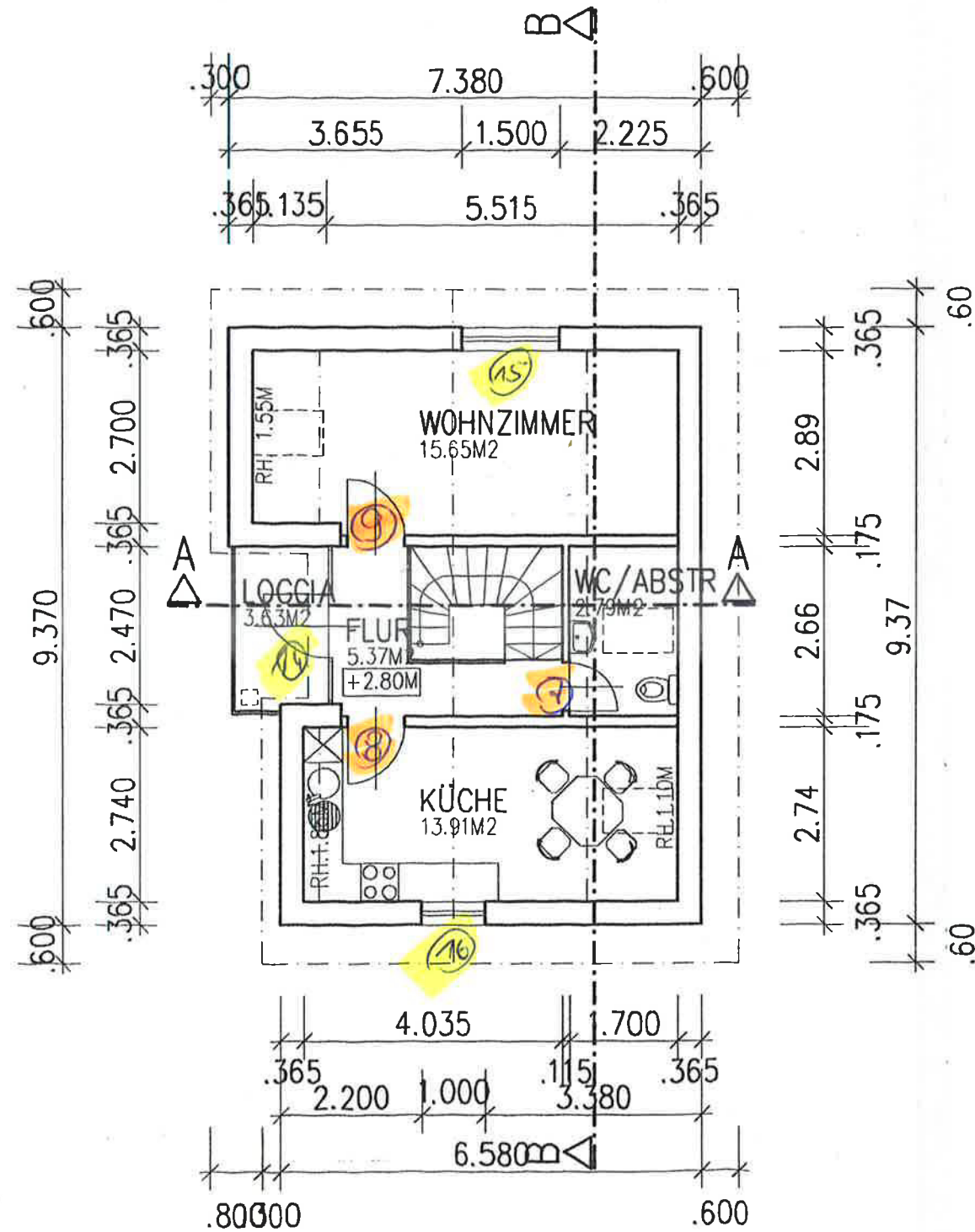
GRUNDRISS DACHGESCHOSS M.1:100
