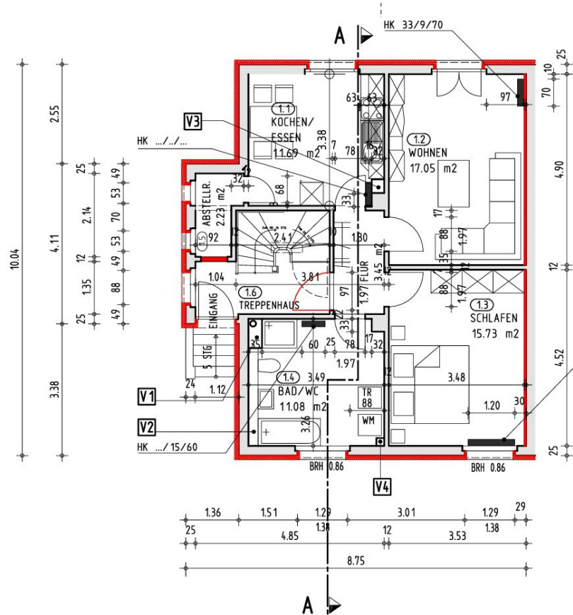
WOHNUNG 1 (ERDGESCHOSS) M. 1:100 WOHNFLÄCHE 61,23 m 2
