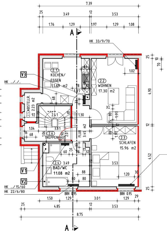
WOHNUNG 2 (OBERGESCHOSS) M. 1:100 WOHNFLÄCHE 61,71 m 2
