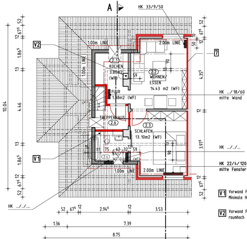
WOHNUNG 3 (DACHGESCHOSS) M. 1:100 WOHNFLÄCHE 36,36 m 2
