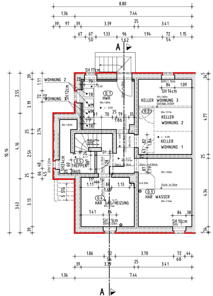
KELLERGESCHOSS M. 1:100
